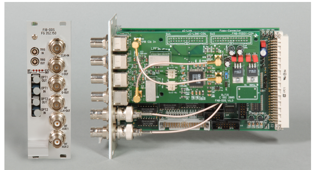
Figure 5: DDS unit.
